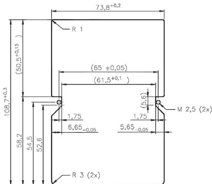
Abbildung 7: Abmessungen Frontplatten-Einbau GPT-4352-60 in mm
